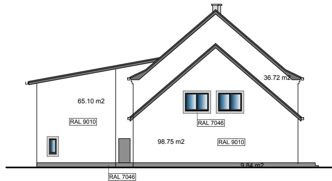
elewacja zachodnia
