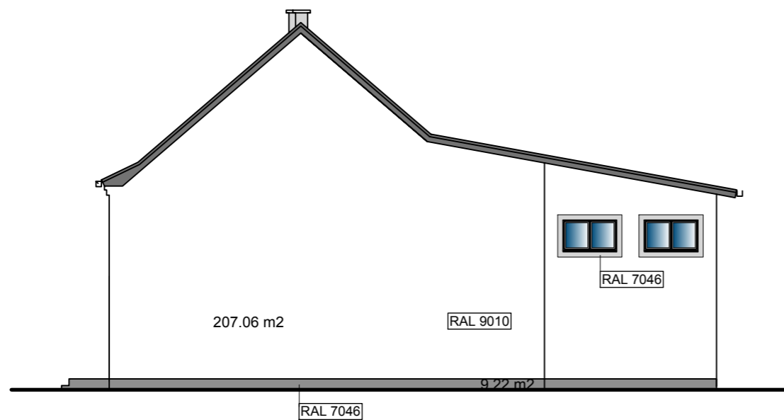
elewacja wschodnia
