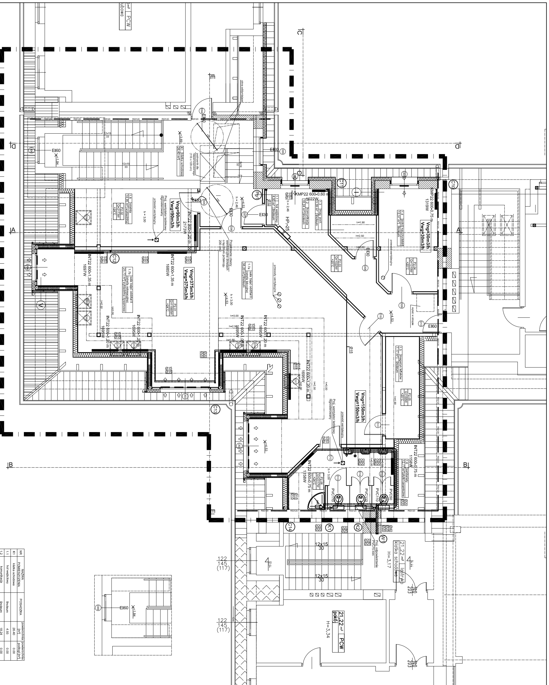
rzut poddasza
