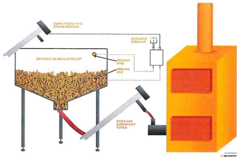
Rysunek 6.6 Kotły na pellet – schemat działania
