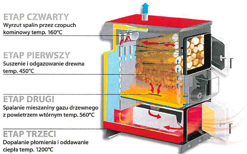
Rysunek 6.8. Zasada działania kotła zgazowującego drewno
