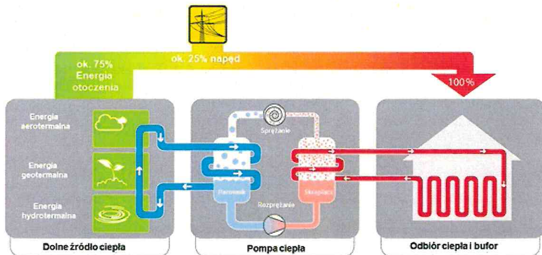
Rysunek 6.4. Zasada działania pompy ciepła
