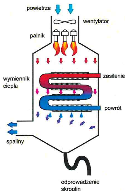
Rysunek 6.3. Schemat funkcjonowania kotła kondensacyjnego
